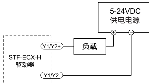
将输出Y1,Y2接成sinking型输出
