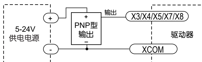
与PNP型输出的连接方式
